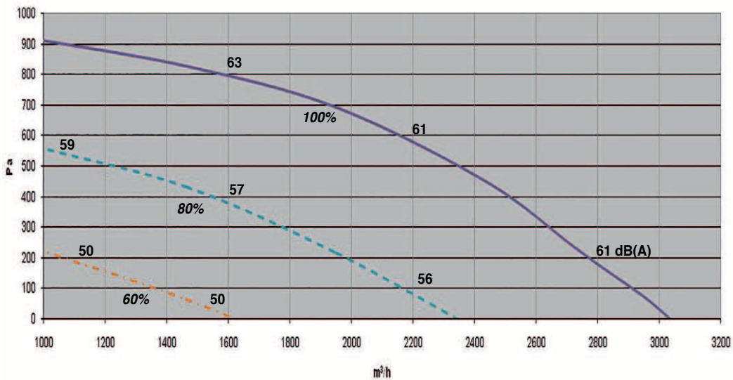
REC PRO 75 - 3800
