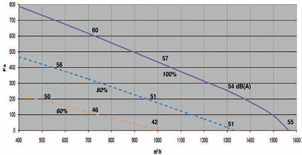
REC PRO 75 - 1300
