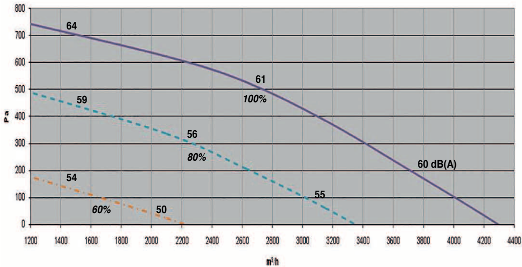
REC PRO 75 - 3800
