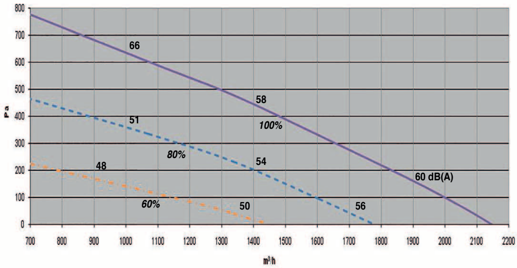
REC PRO 75 - 2800
