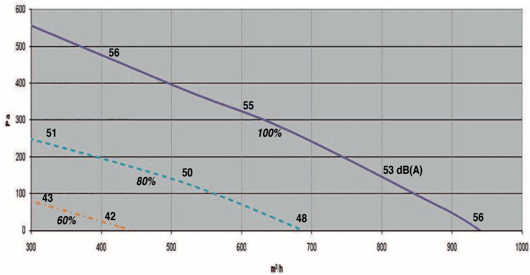
REC PRO 75 - 1300
